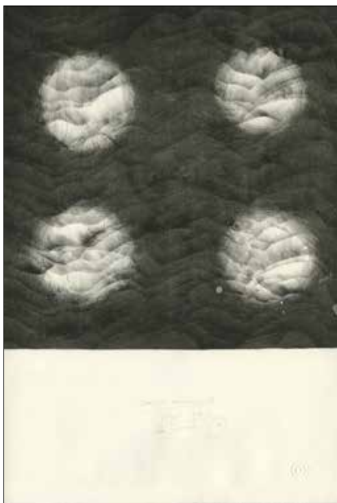
Schemat randomizacji-09|74×51|litografia|2018
